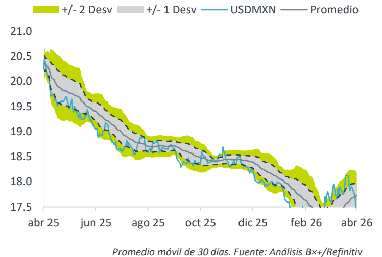
USDMXN
