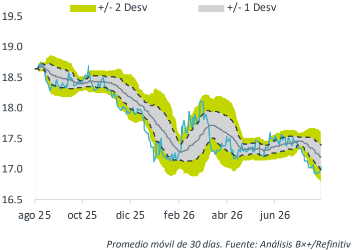
USDMXN
